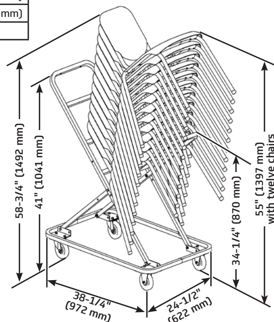
Move 'N Store Cart
